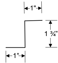
Z TRIM
