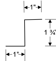
Z TRIM
